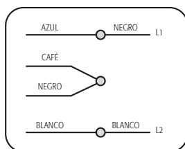
Conexión a 220 V~
