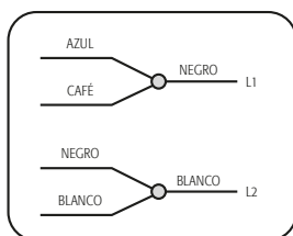
Conexión a 127 V~
